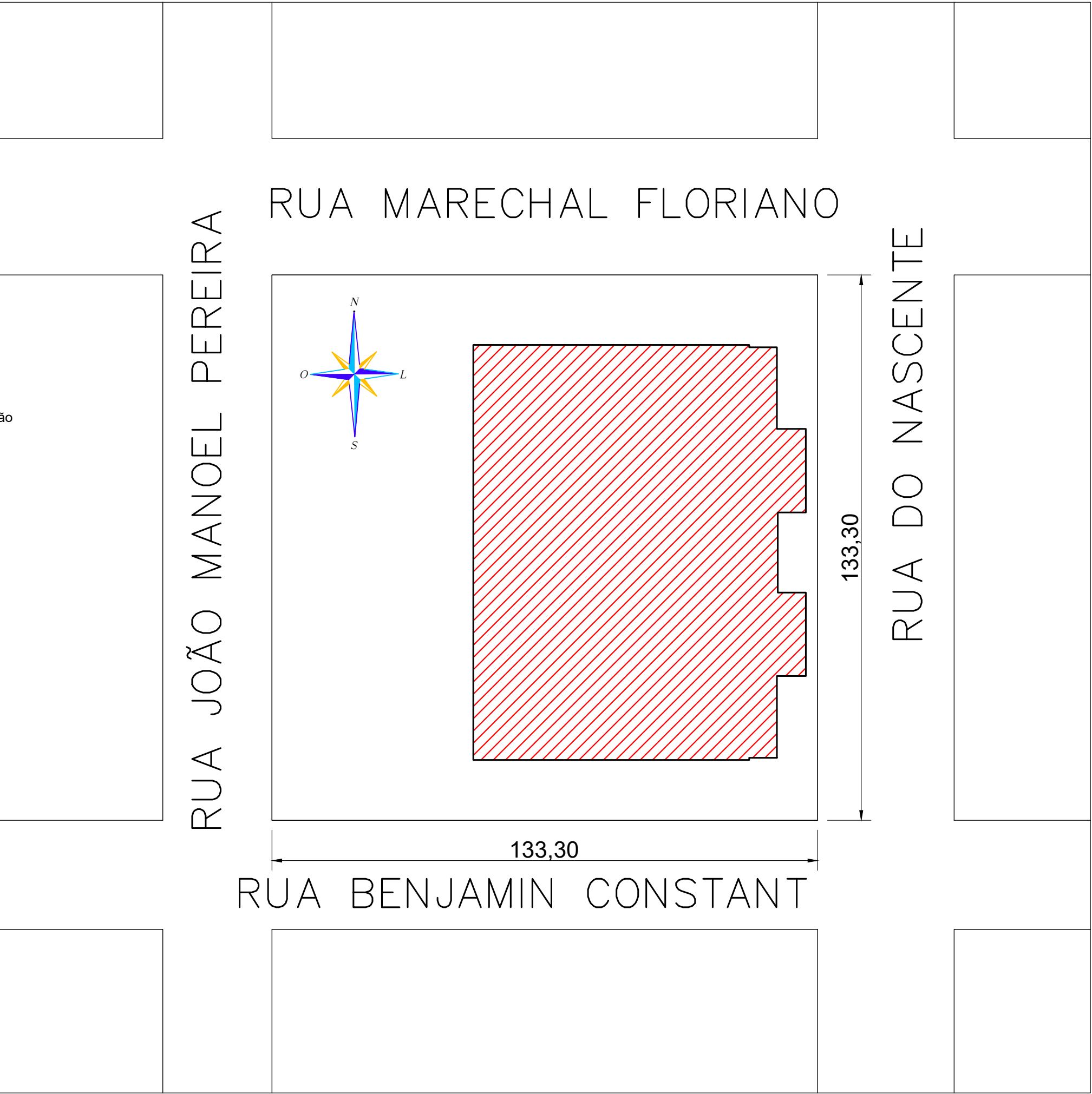
Planta de Situação ESCALA: = 1:750
