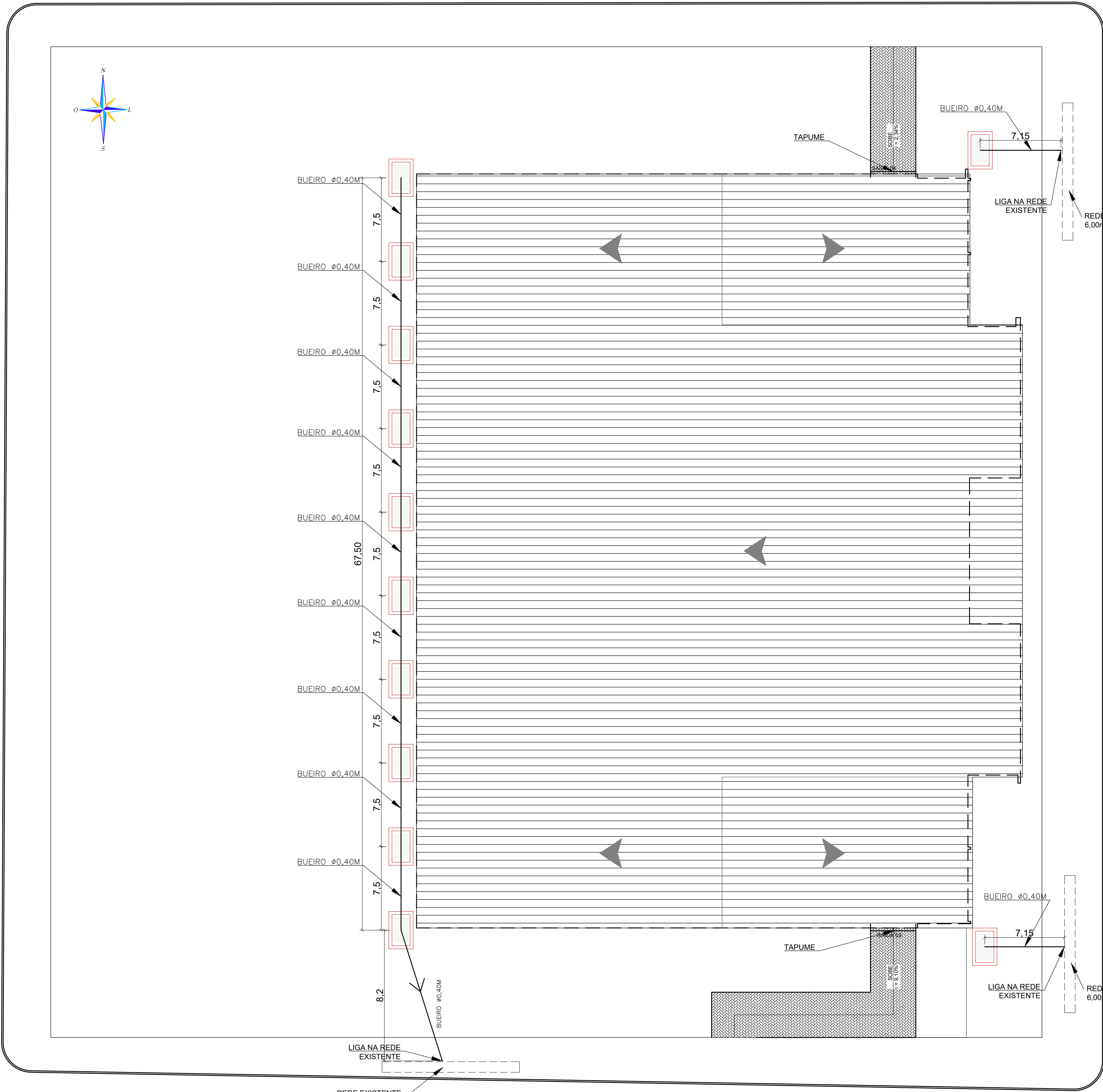
Planta de Localização / Drenagem ESCALA: = 1:250
